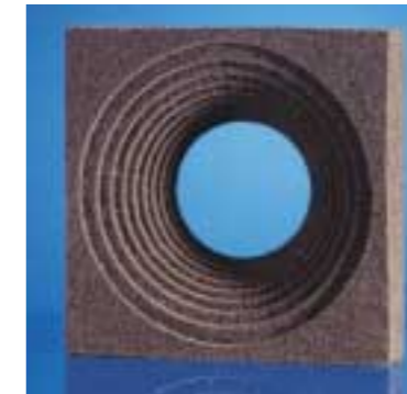
Millimetergenaue Maßarbeit: Die Hochtönerschallführung aus lasergeschnittenen Filzelementen.
