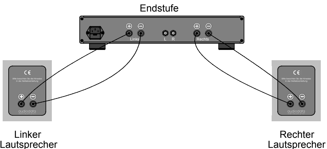
Zeichnung 1.2.1: Lautsprecheranschluß mit Single-Wiring Lautsprecherkabel
