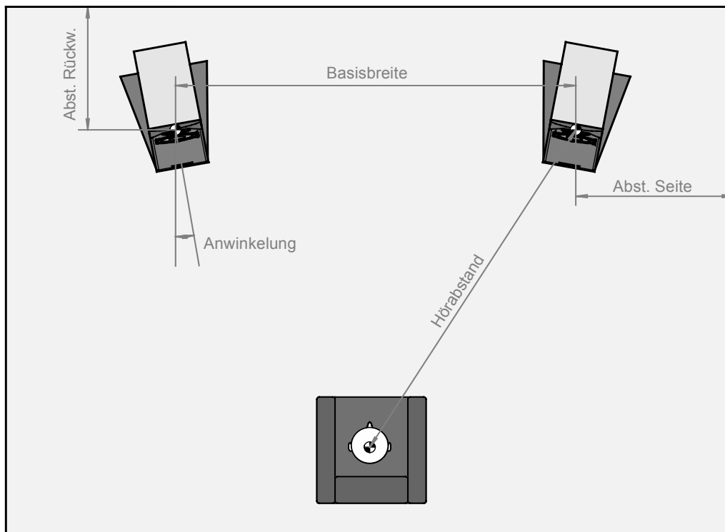
Zeichnung 2.2.1: Hörraum aus der Vogelperspektive (Beispiel Echelle ) zur Begriffsdefinition
