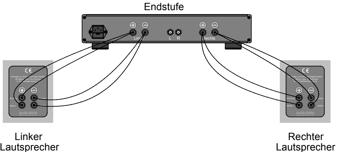
Zeichnung 1.2.3: Lautsprecheranschluß mit Bi-Wiring Lautsprecherkabel
