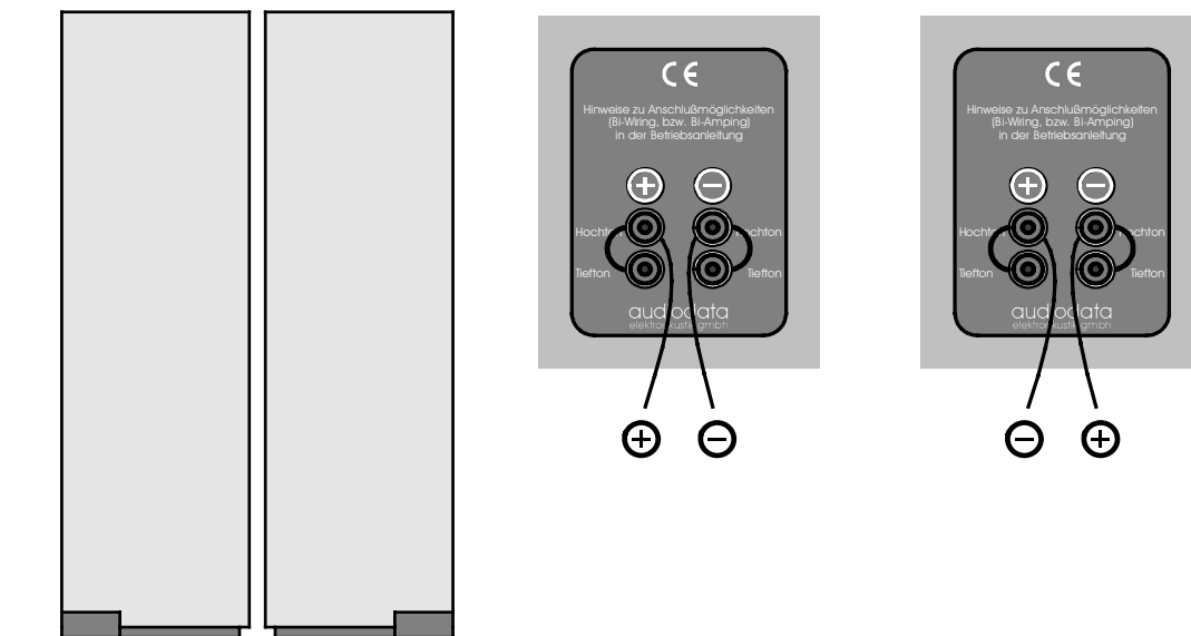
Zeichnung 2.1.1: Lautsprecherposition und Anschlußweise beim Power-Einspielen
